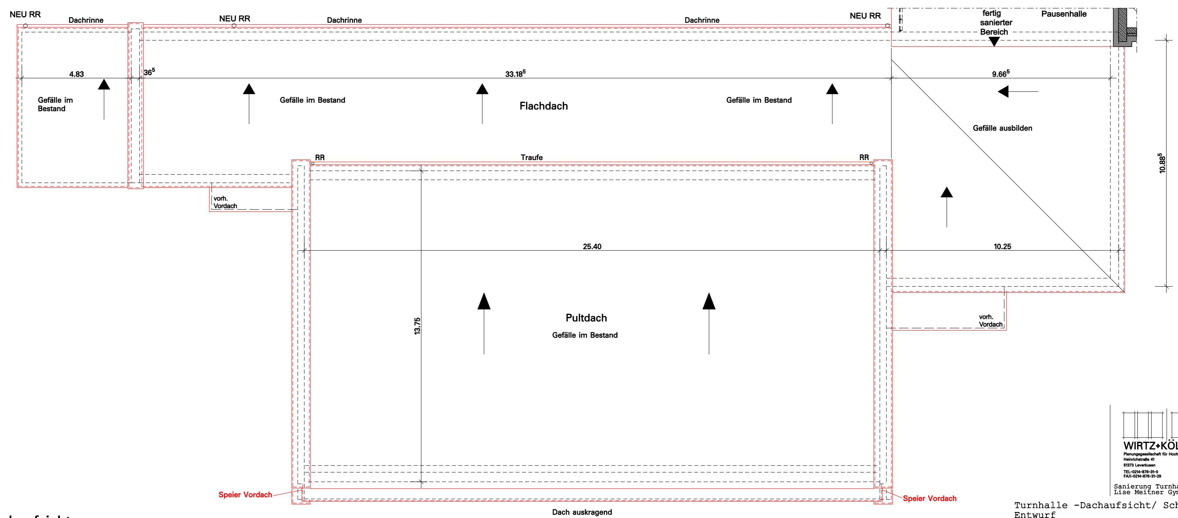
Dachaufsicht
