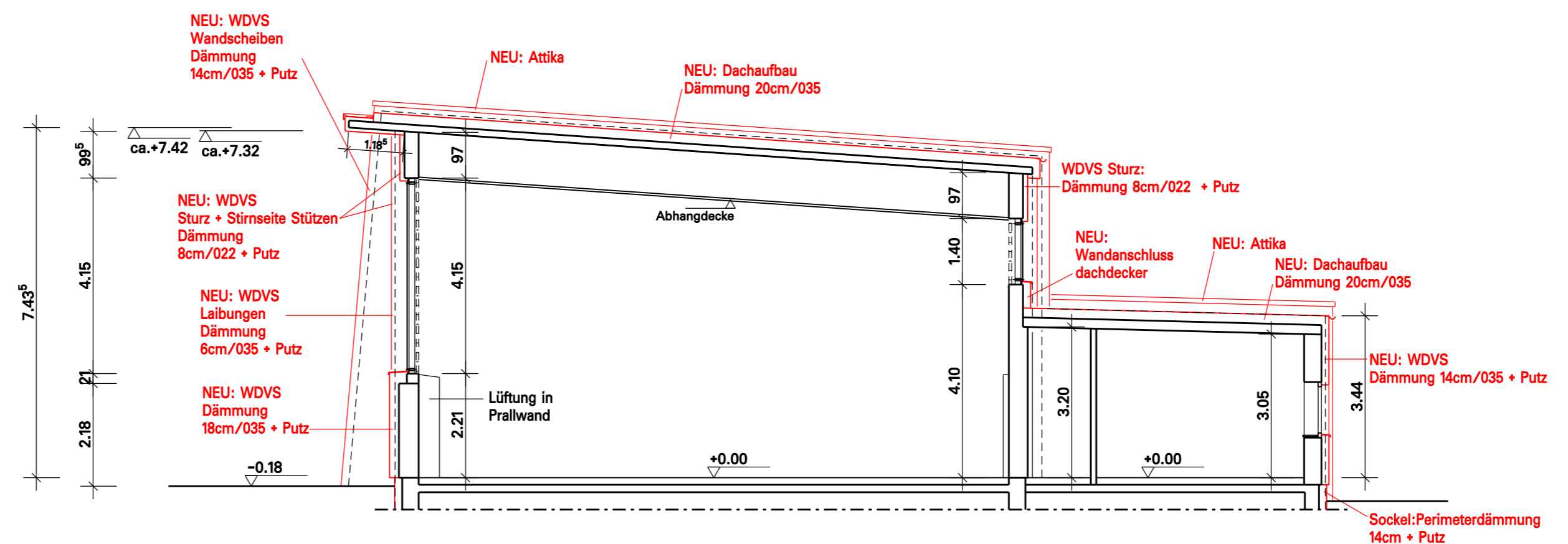
Schnitt Entwurf
