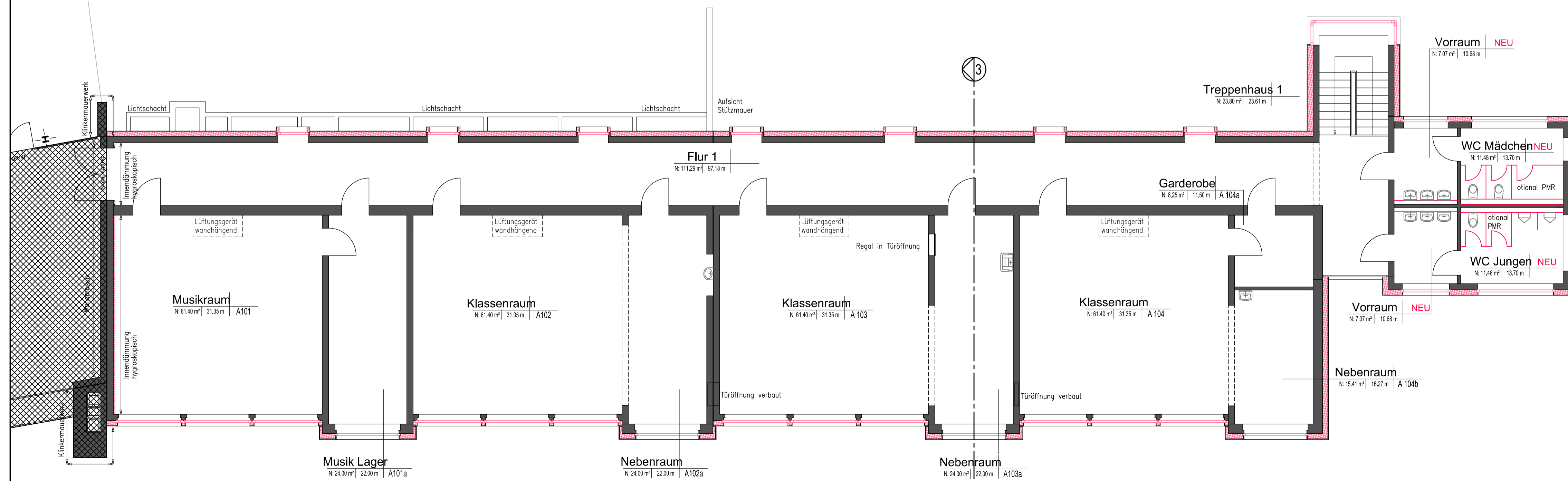
Trakt A | 1.Obergeschoss
