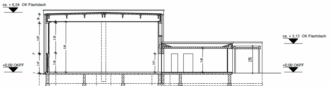
Schnitt A-A
