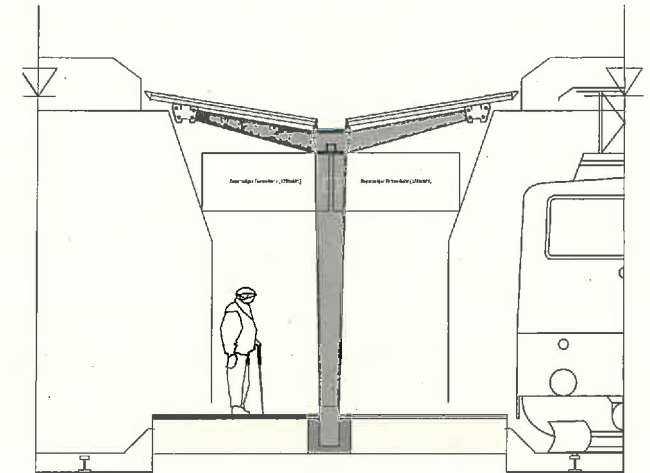
Systemdach Zwiesel - einstielig
