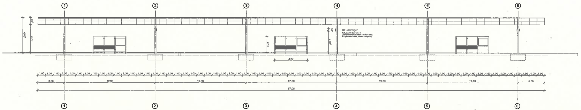
Längsschnitt ZOB-Überdachung
