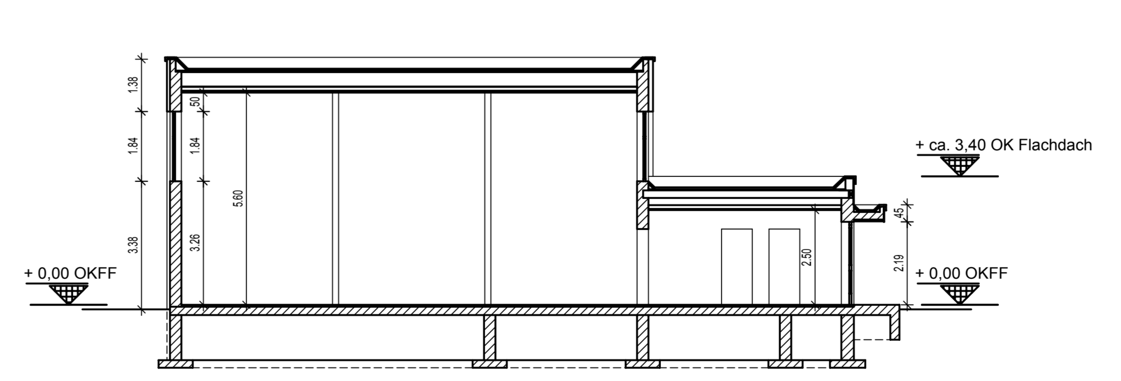
Schnitt H-H
