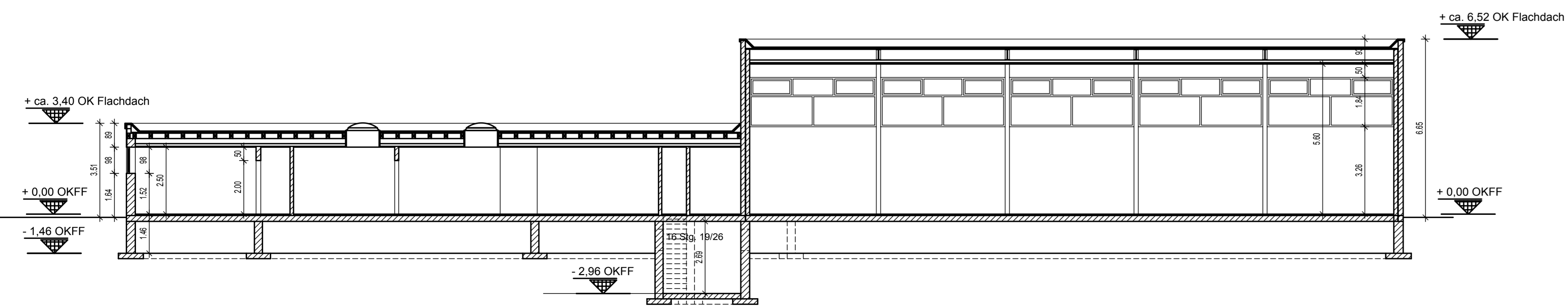
Schnitt G-G
