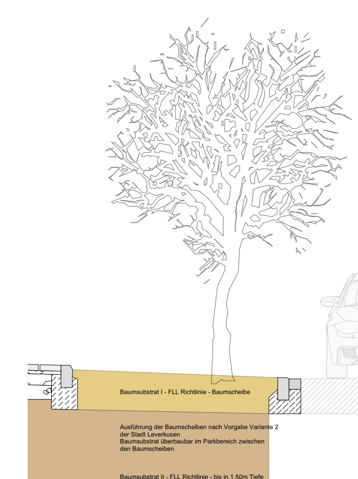
5 SCHNITT - BAUMSCHEIBE 3 - M 1:50 012 DW 03 EG GR 001 00 -
