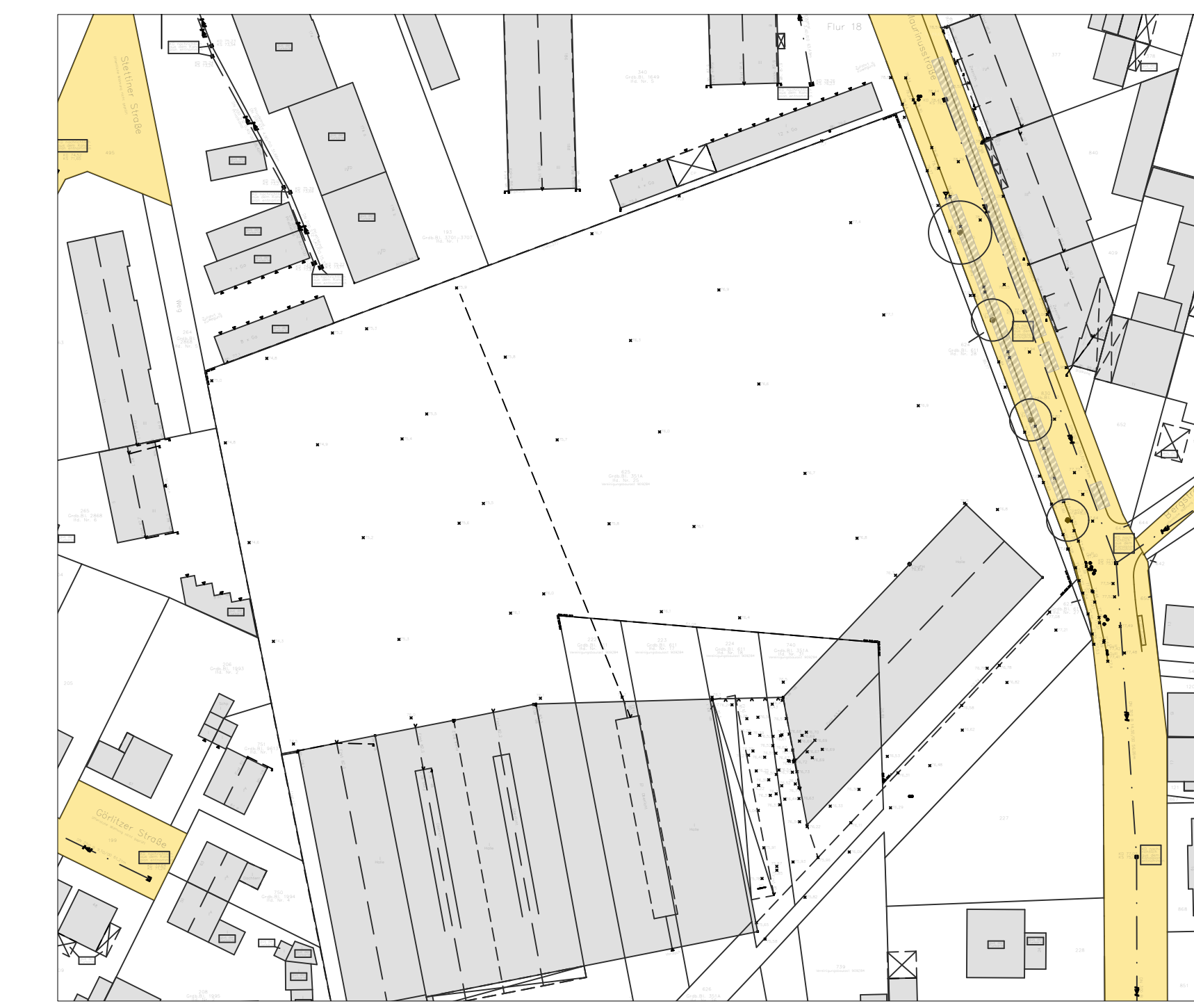
2 ÜBERSICHTSPLAN BESTAND - M 1:1000 012 DW 03 EG GR 001 00 -
