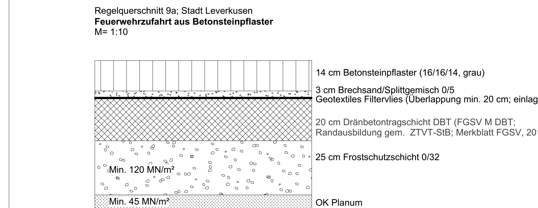
3 REGELQUERSCHNITTE - STADT LEVERKUSEN 012 DW 03 EG GR 001 00 -
