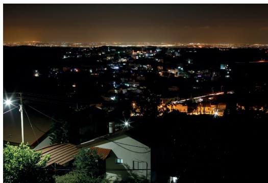
Abbildung 1.5 Nächtliche künstliche Beleuchtung durch Straßenlaternen, erleuchtete Gebäude, Leuchtreklame und Fahrzeugbeleuchtung führt zu einem hellen Himmelsleuchten. Das Bild wurde vom wesentlich geringer beleuchteten Westjordanland in Richtung Israel aufgenommen (© J. RYDELL).
