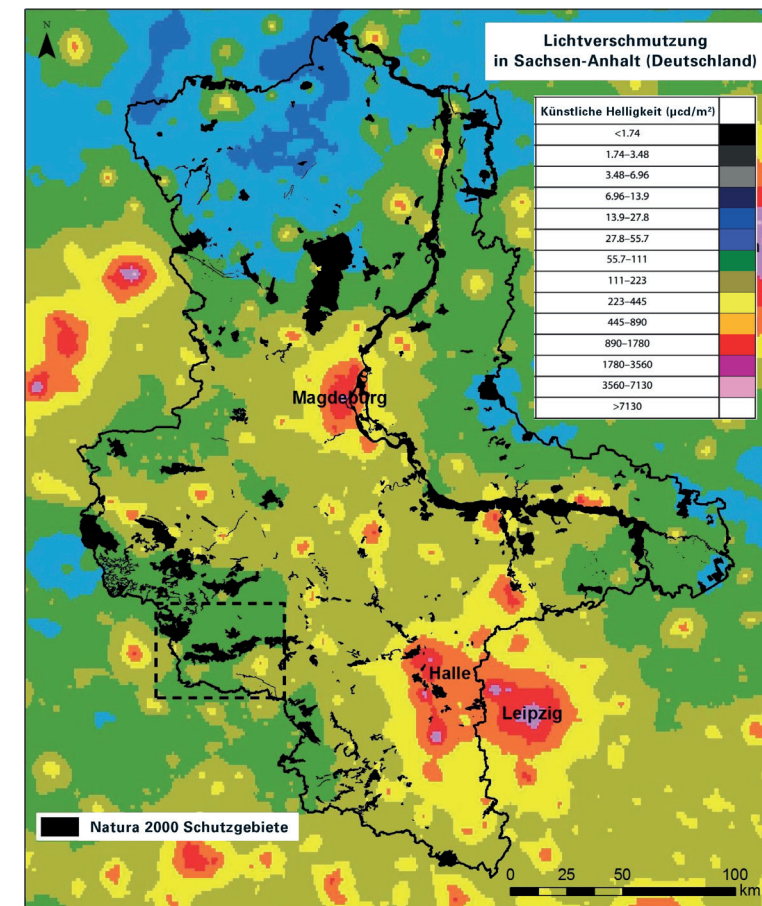
Abbildung 3.1 Karte von Sachsen-Anhalt in Deutschland mit Natura 2000 Gebieten und nächtlichem Kunstlicht zur Lokalisierung potenzieller Konflikte zwischen Lichtverschmutzung und geschützten Fleder- mauslebensräumen. Die gestrichelte Linie zeigt den Bereich von Abbildung 3.2 (© K. KUHRING & M. FRITZE, Quelle GIS-Layer: F. FALCHI).
