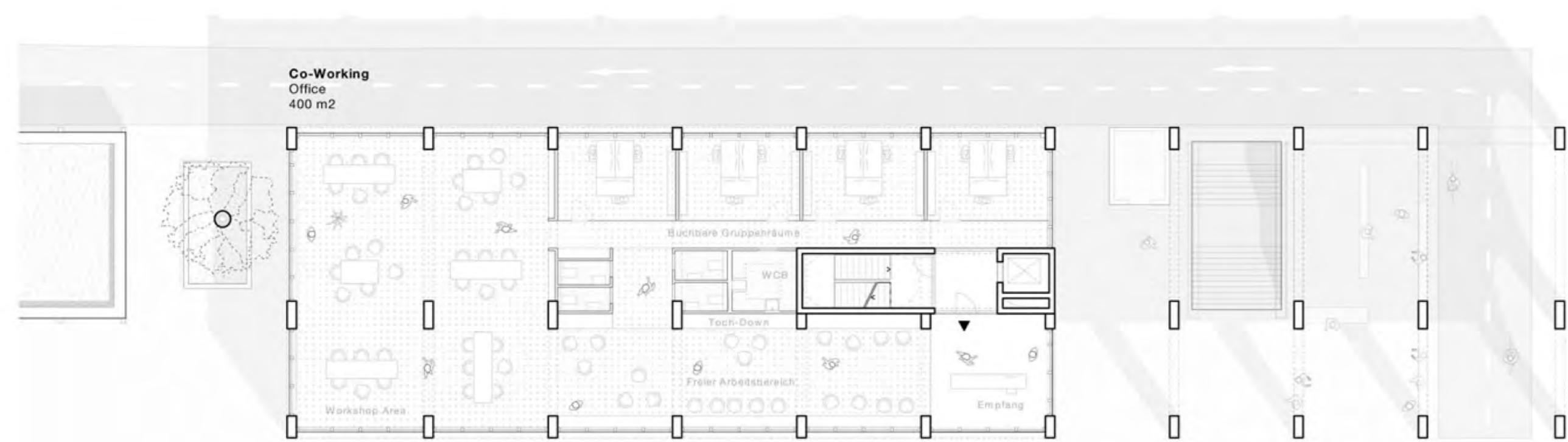
Erdgeschoss M 1:200
