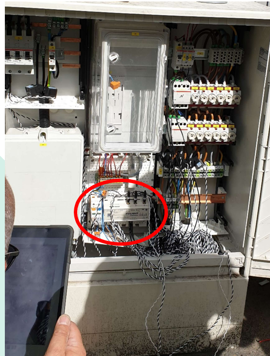
Umbau eines Schaltschranks mit neuem Rundsteuergerät (Testinstallation)
