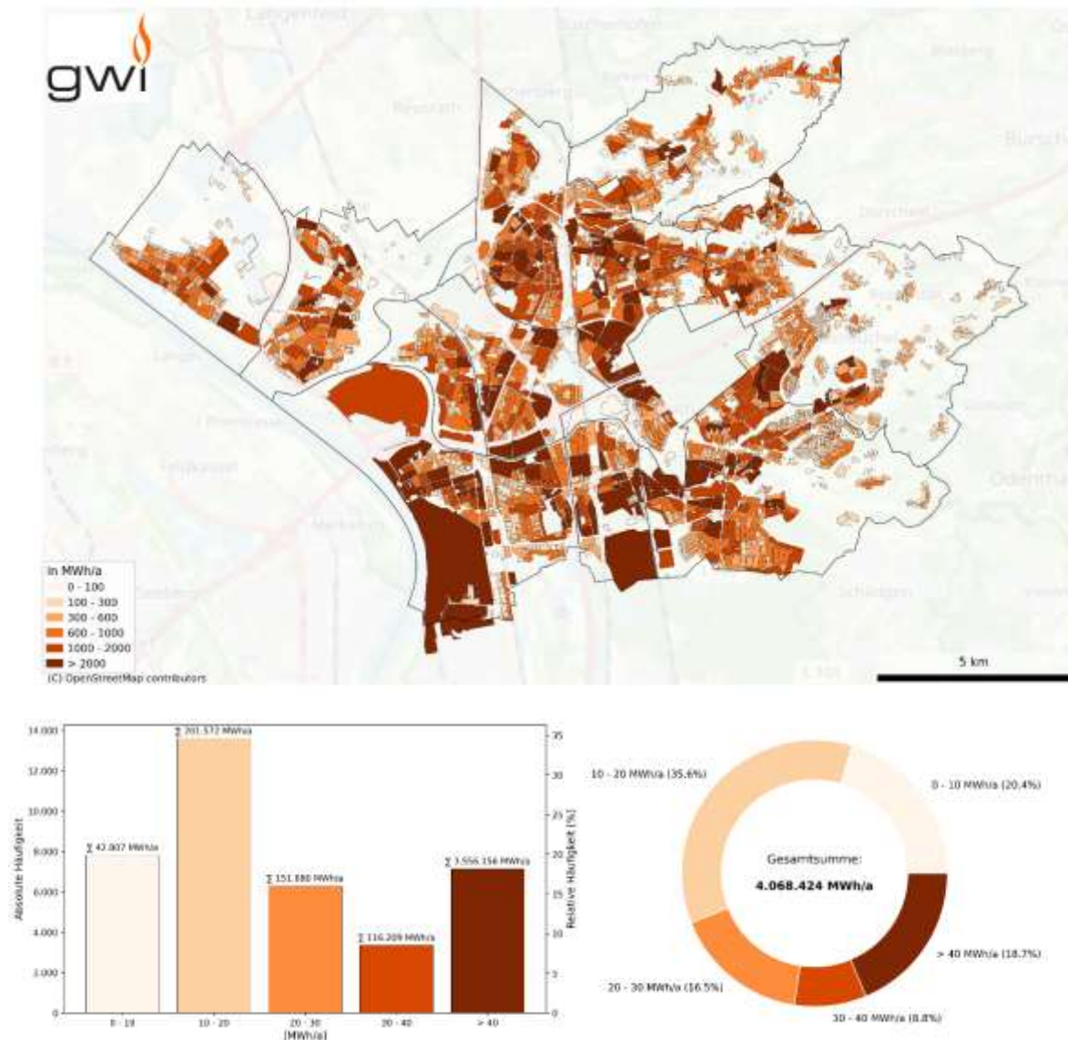
Abbildung 38: Endenergiebedarfe im Baublöck sowie deren statistische Verteilung auf Gebäudeebene
