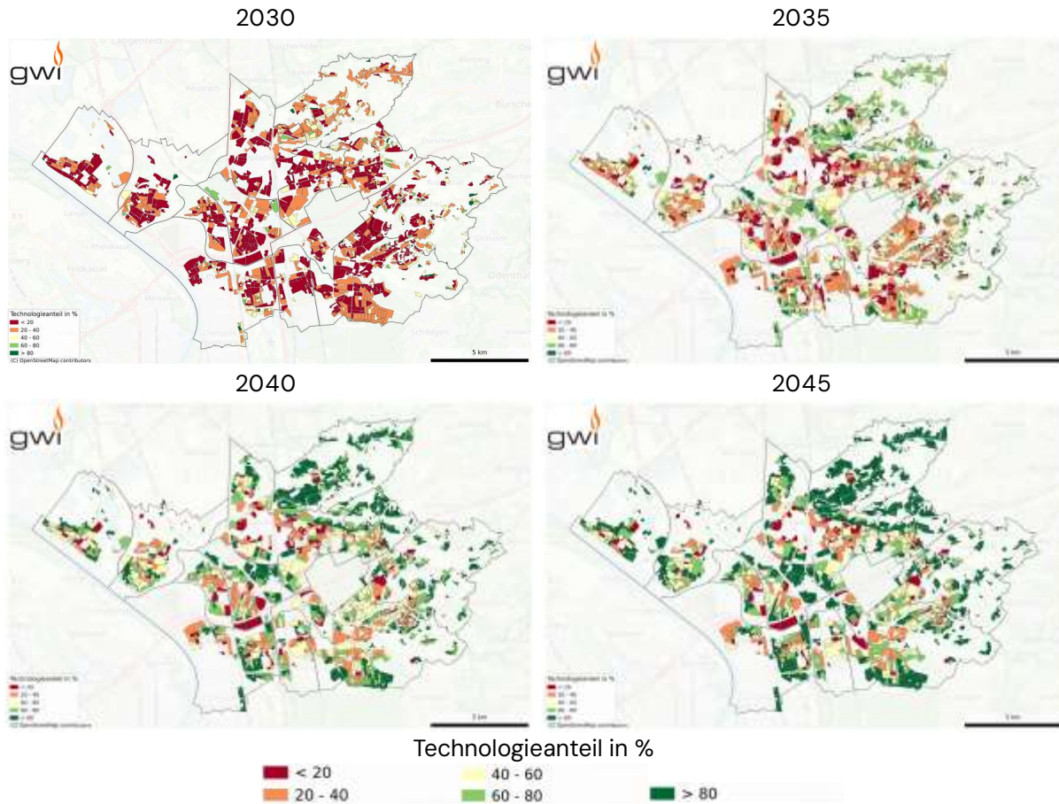
Abbildung 68: Wärmepumpen im maßgeblichen Zielszenario als Technologieanteil Wärmepumpe. Baublöcke mit ausschließlich industrieller Nutzung wurden nicht berücksichtigt
