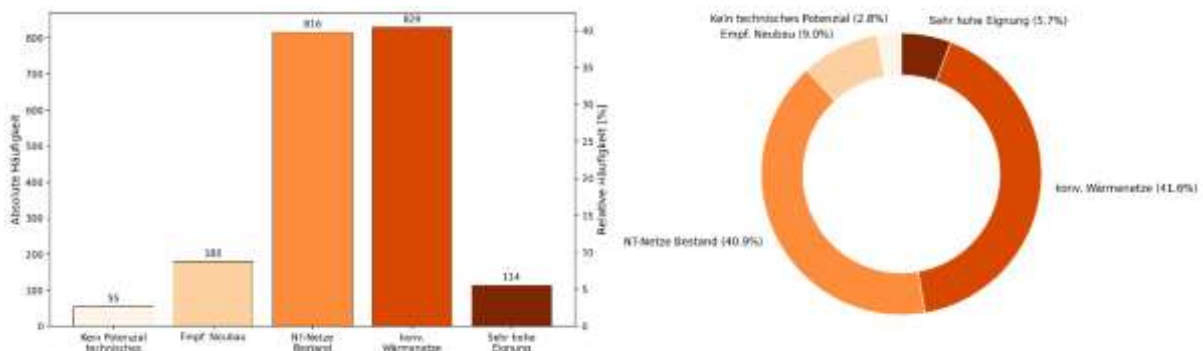
Abbildung 47: Eignungsklassifikation der Baublöcke nach KEA-BW inkl. Bestandsnetze (grün) sowie statistische Verteilung der Baublöcke
