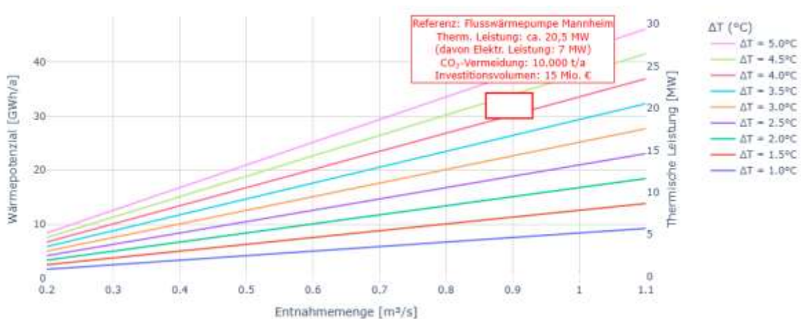
Abbildung 58: Wärmepotenzial und Wärmeleistung in Abhängigkeit der Entnahmemenge bei verschiedenen Temperaturdifferenzen des Entnahmewassers
