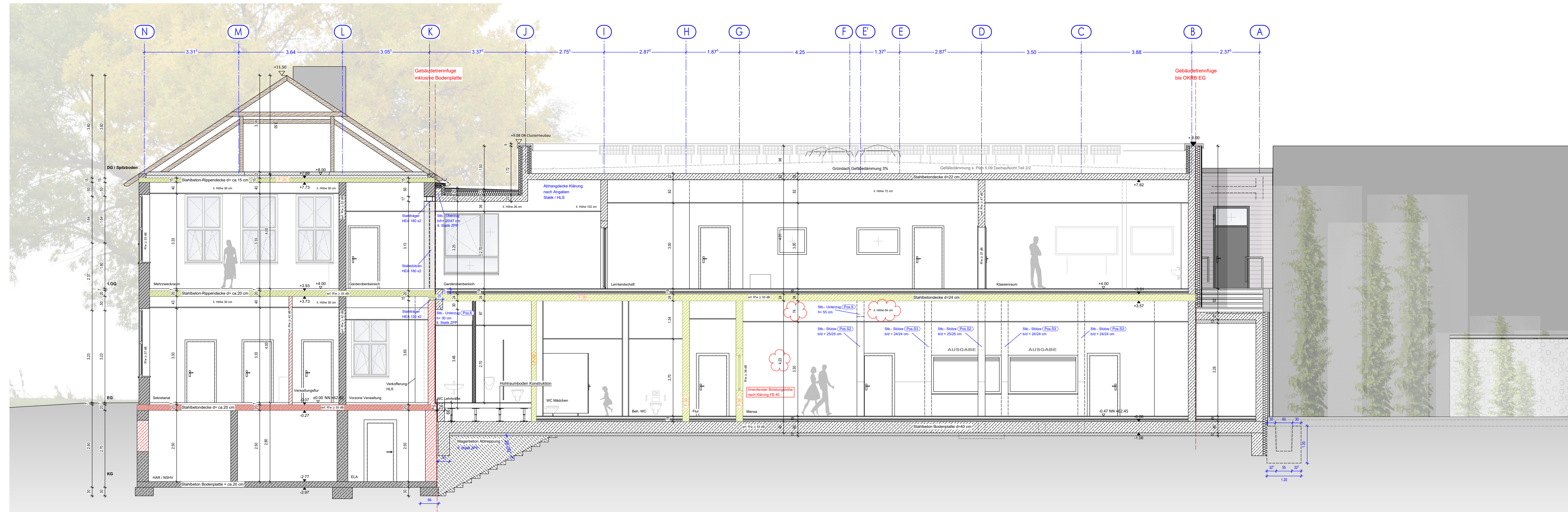
Schnitt D-D
