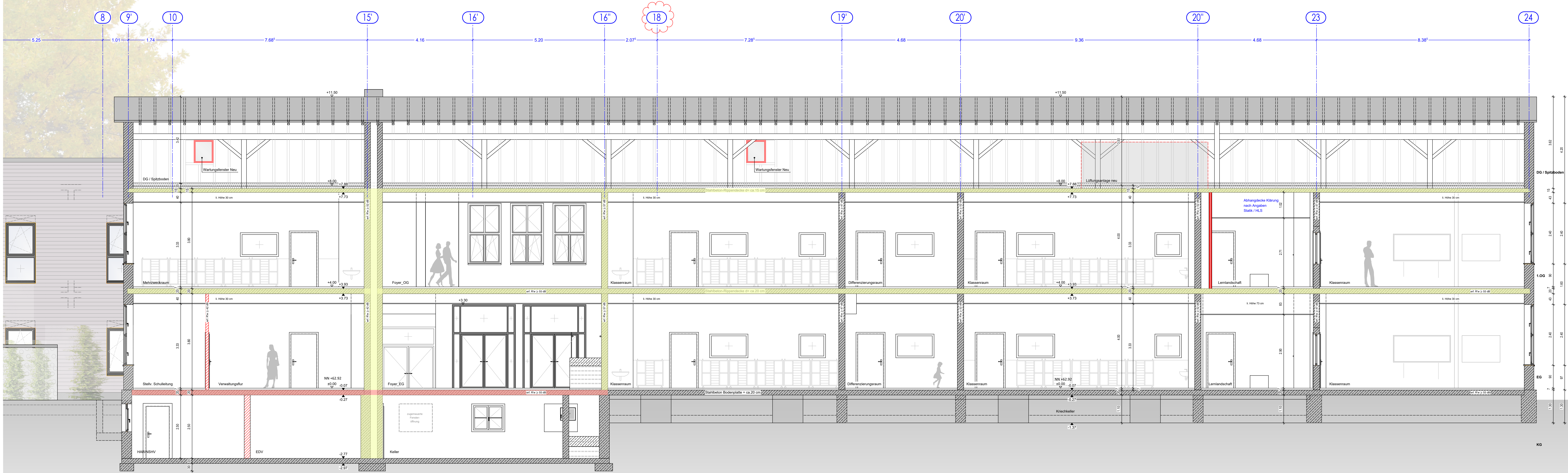
Schnitt B-B
