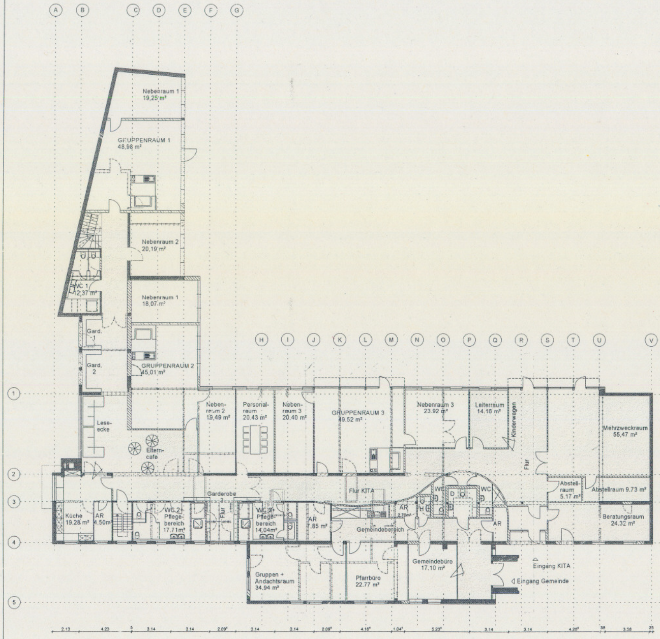
Grundriss EG Neuplanung Variante B
