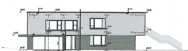
Ansicht / Schnitt Westen
