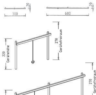
78035 Sandtransport, 3 m lang 78036 Sandtransport, 6 m lang
