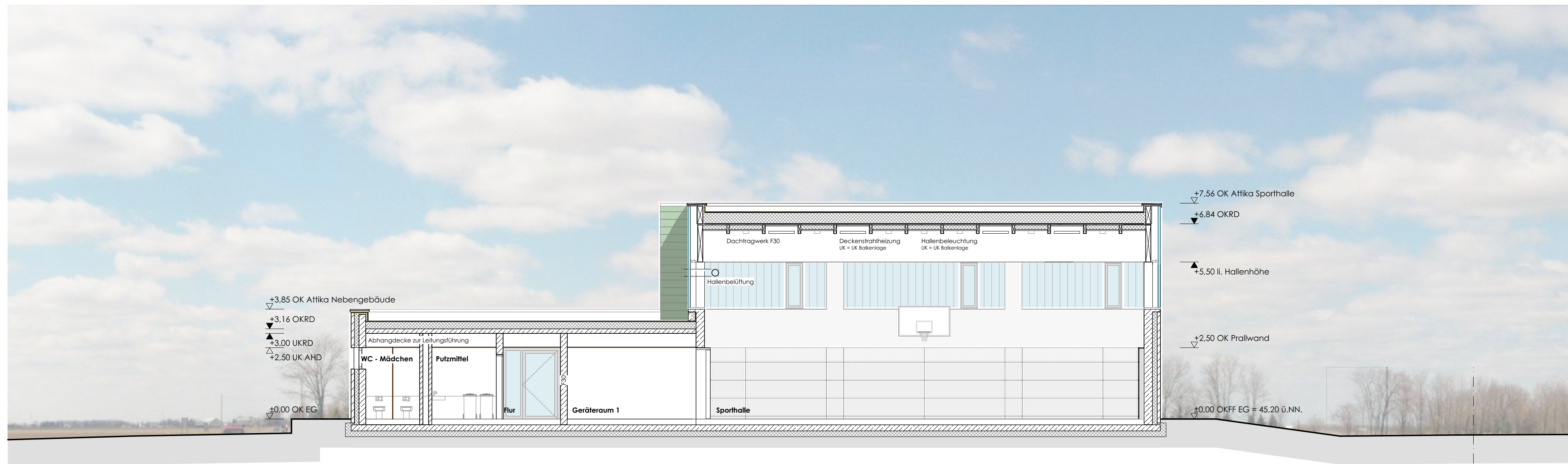
SPORTHALLE GGS LÖWENZAHN SYSTEMSCHNITT AA 1:100
