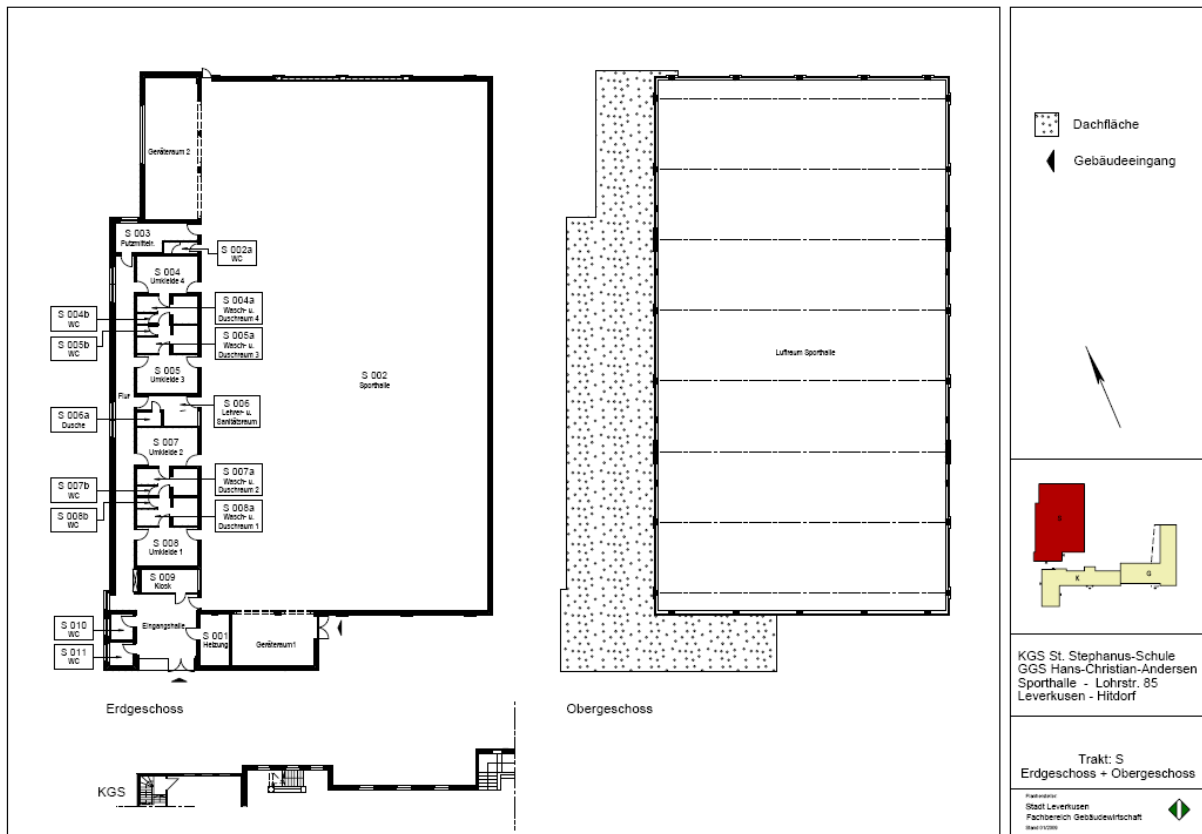
Grundriss Sporthalle GGS/KGS Lohrstraße
